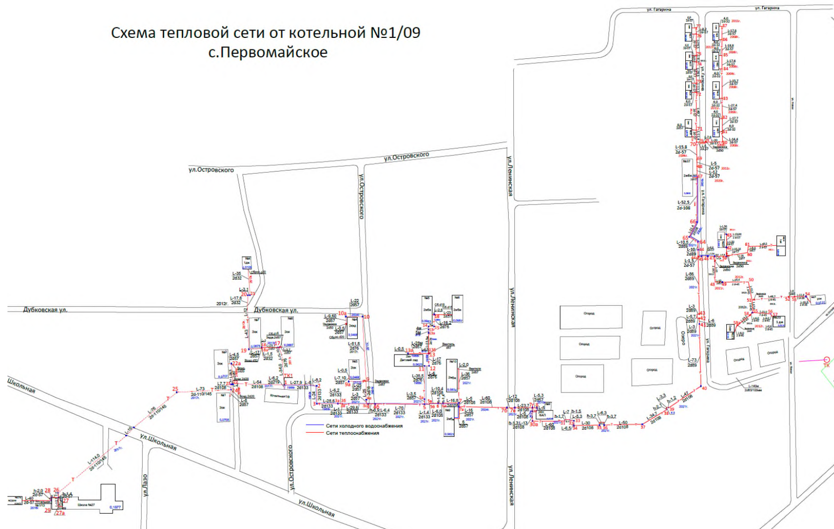
Рис. 2.3 – Схема теплоснабжения села Первомайское от котельной № 1/9
