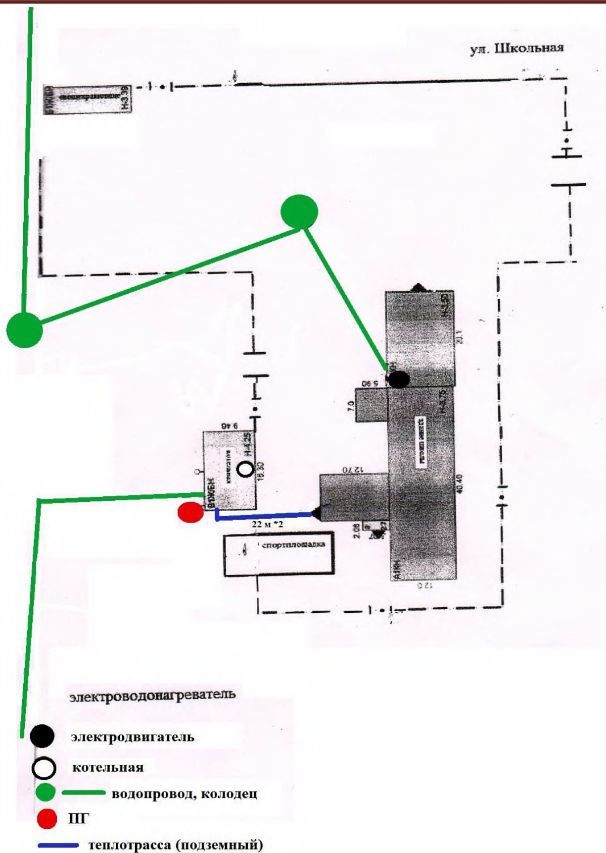
Рис. 2.4 – Схема теплоснабжения села Первомайское от котельной КГБУ Первомайской КШИ
