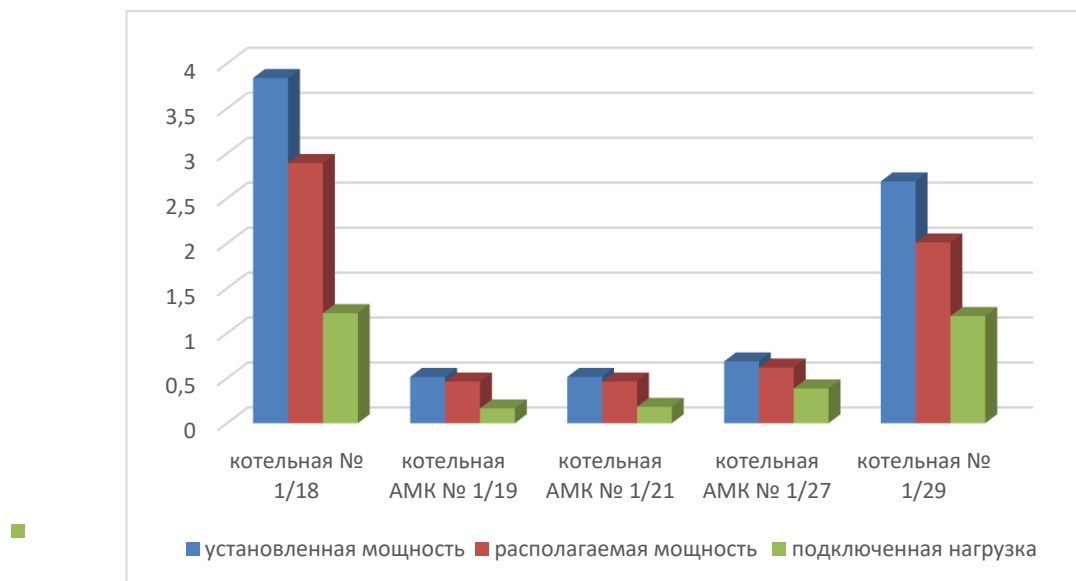
Рис. 1.3 – Распределение мощностей источников тепловой энергии
