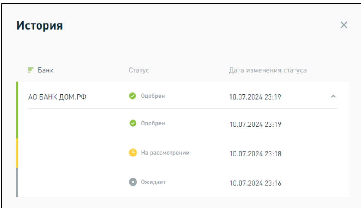
Рисунок 64 – История одобрения
