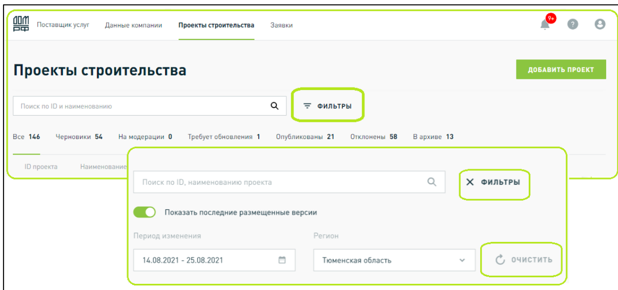
Рисунок 10 – Фильтры
