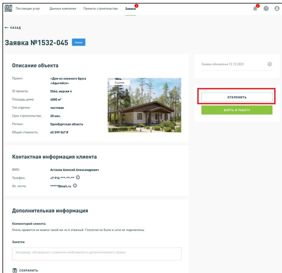
Рисунок 107 – Кнопка «Отклонить»
