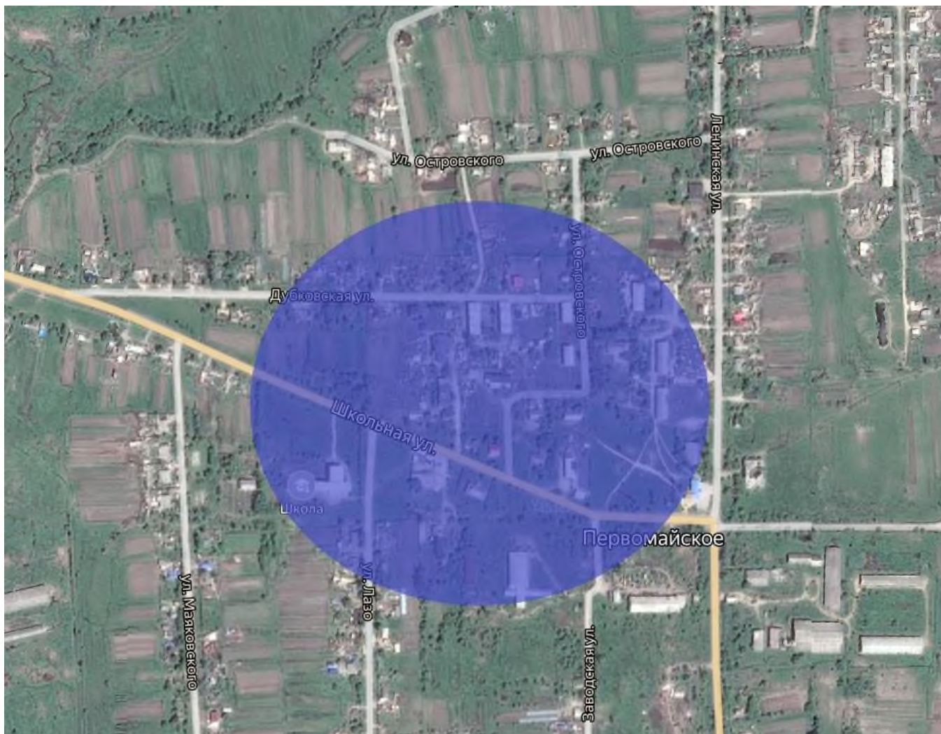
Рис. 2.1 – Зона действия теплоснабжения котельной № 1/9 села Первомайское
