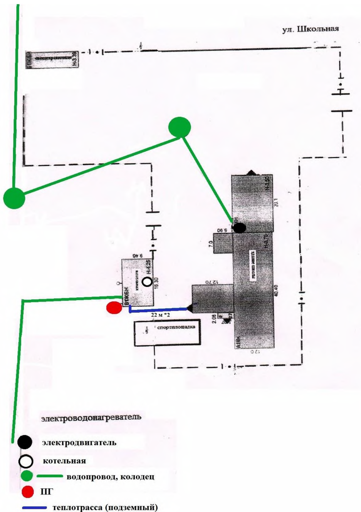
Рис. 2.5 – Схема теплоснабжения села Первомайское от котельной КГОБУ Первомайской КШИ
