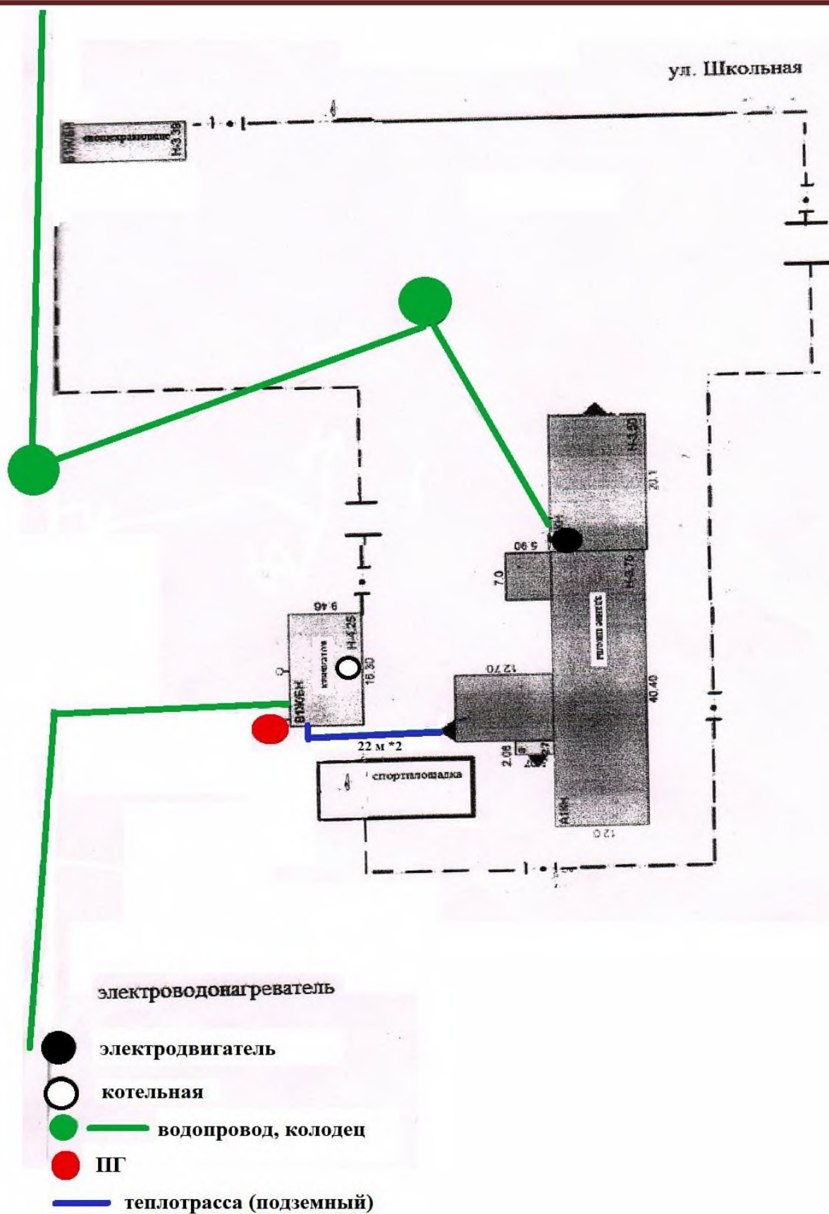
Рис. 2.4 – Схема теплоснабжения села Первомайское от котельной КГОБУ Первомайской КШИ
